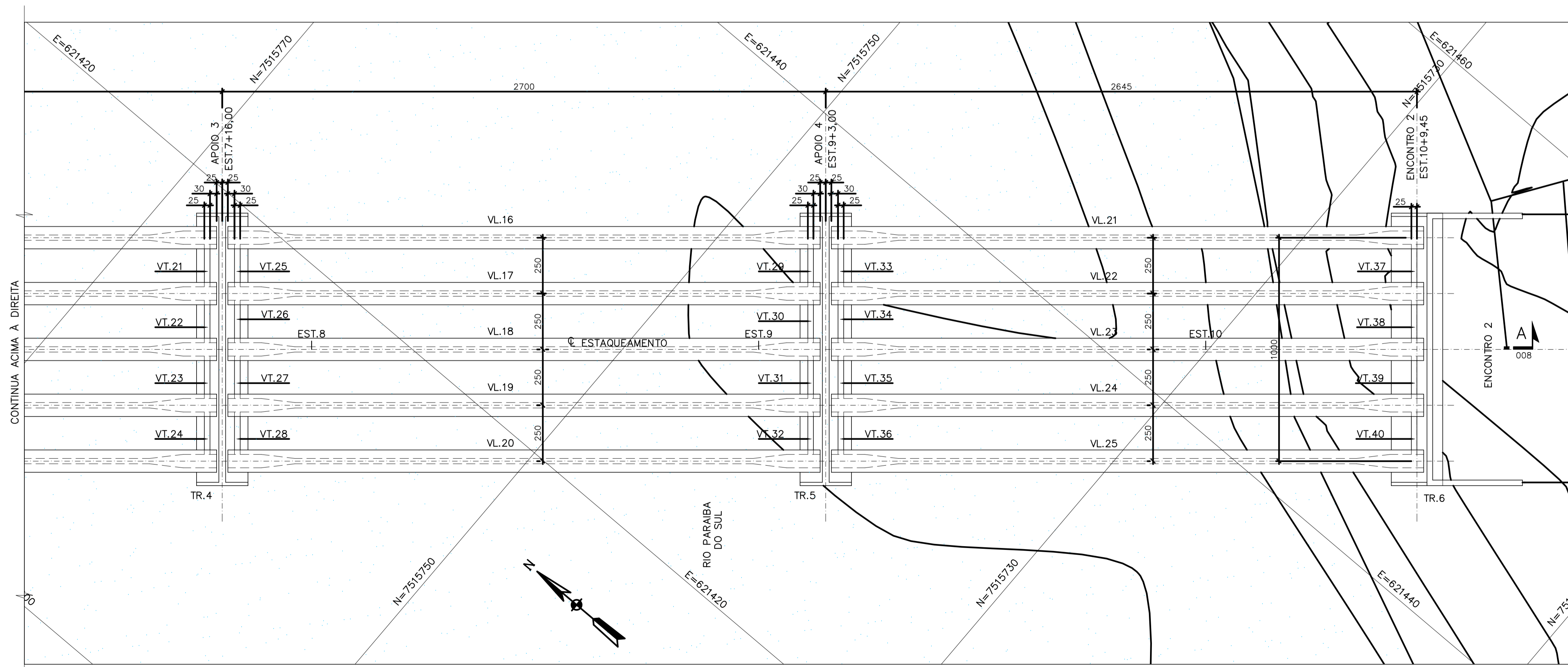
LOCAÇÃO DAS VIGAS PRÉ MOLDADAS - PLANTA - 2ª PARTE ESC 1:125
